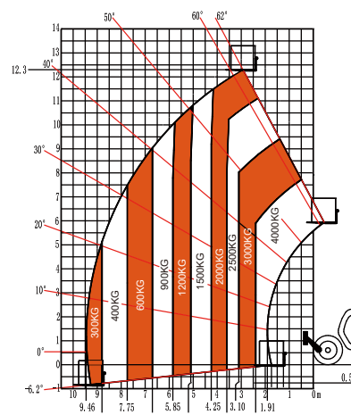
Гидравлические выносные опоры полностью разложены
