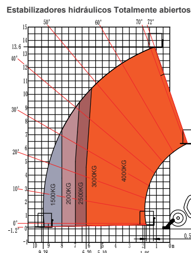
DIAGRAMA DE CARGA PARA TERRENO DIFÍCIL Estabilizadores hidráulicos Totalmente abiertos
