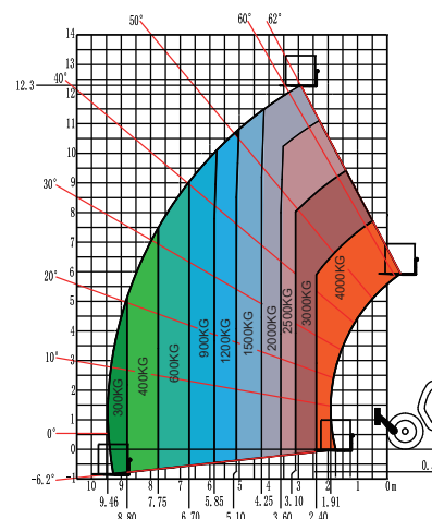
DIAGRAMA DE CARGA PARA TERRENO DIFÍCIL Estabilizadores hidráulicos Totalmente abiertos
