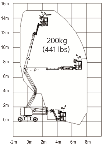
Courbe de travail du modèle A13JE
